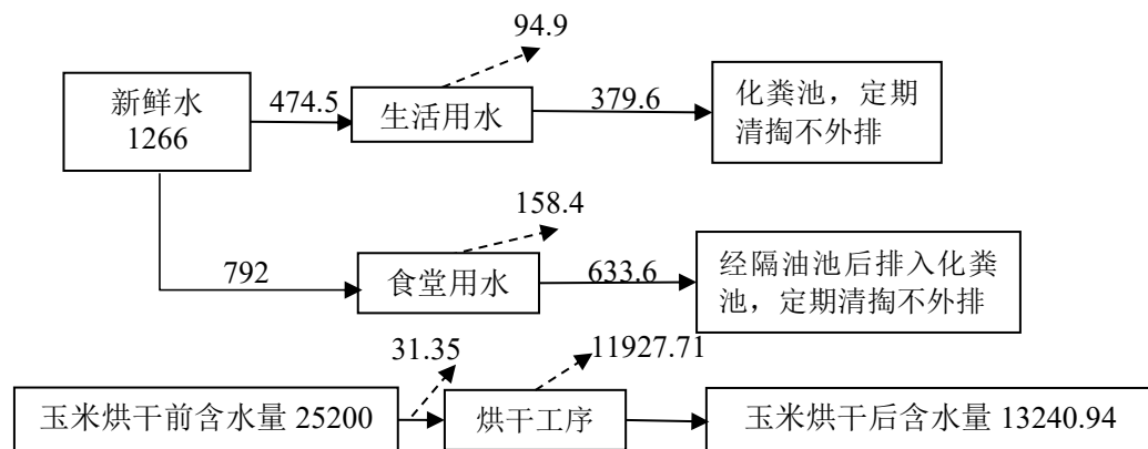
图 2-2 项目水量平衡图 单位:m³/a
