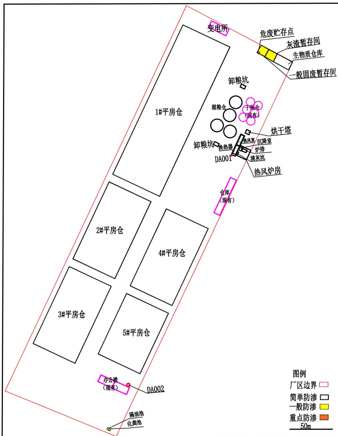
附图 3 厂区分区防渗图
