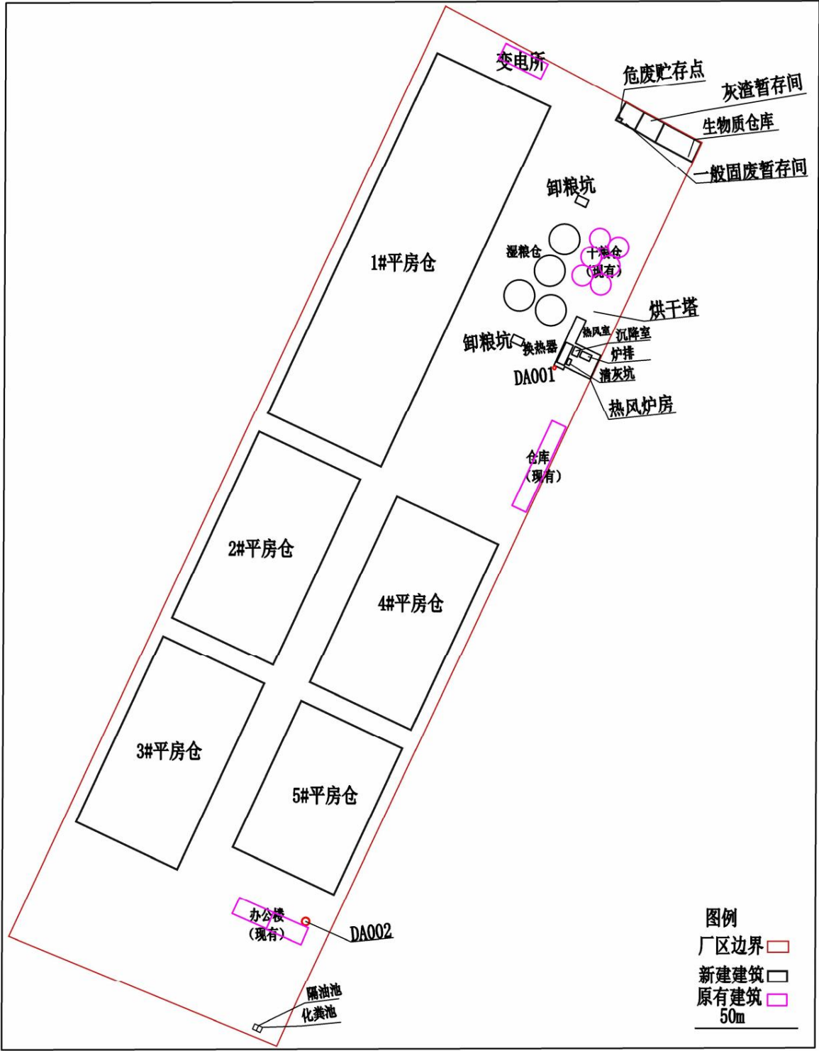
附图 2 厂区平面布置示意图
